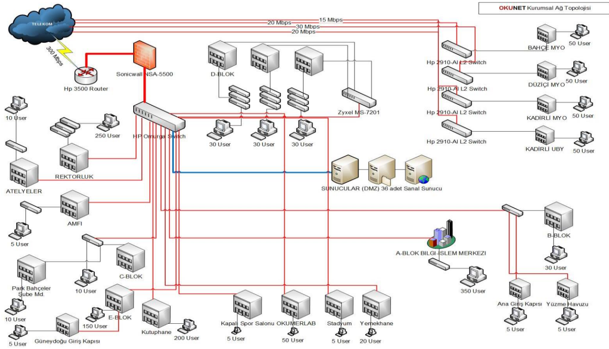
Şekil 1: Osmaniye Korkut Ata Üniversitesi Ağ Planı
