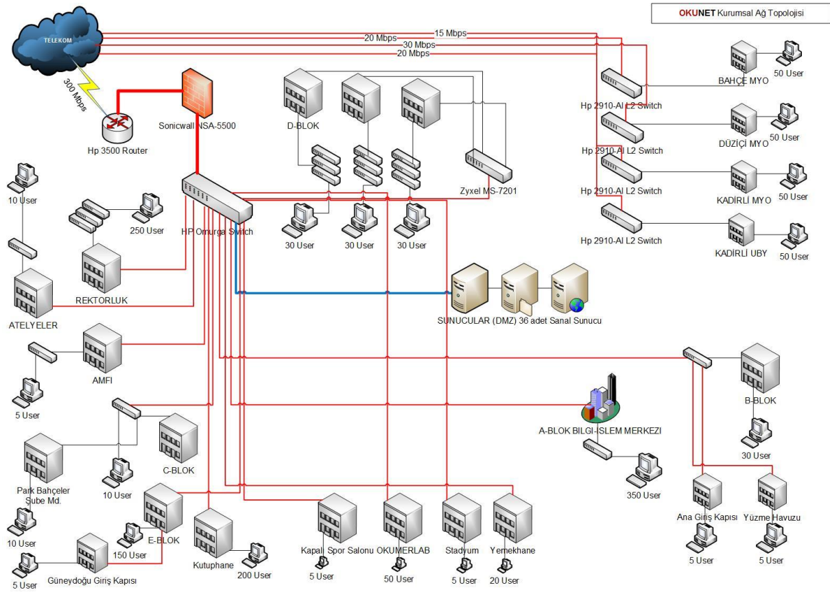
Şekil 3: Osmaniye Korkut Ata Üniversitesi Ağ Planı
